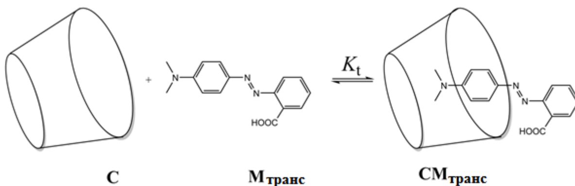
Рис. 2 – Образование комплекса включения СМ транс .
