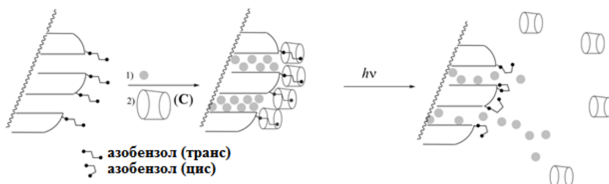
Рис. 5 – Разрушение комплекса включения азобензол-циклодекстрин, вызванное фотоизомеризацией, для доставки красителя (показанного в виде серых кружков).
