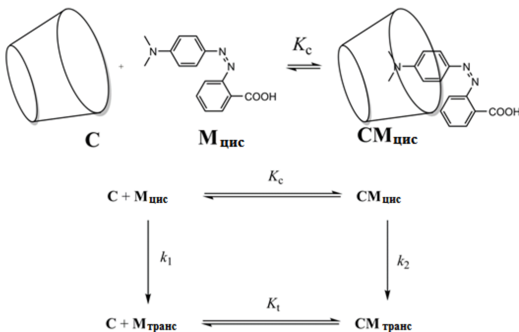
Рис. 4 – Кинетическая схема изомеризации М_{цис} в присутствии С .
