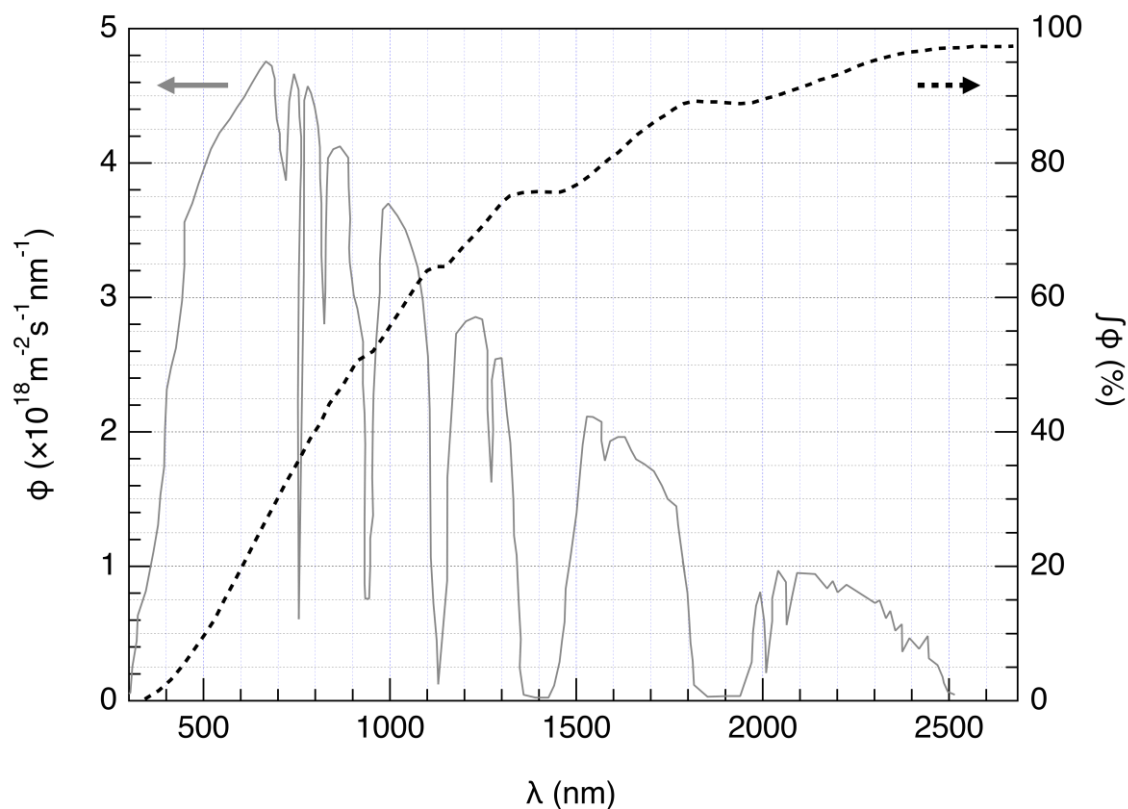
Abb. 3 – Linke Achse: Solarer Photonenfluss \phi . Der Photonenfluss ist die Anzahl an Photonen, welche pro Fläche und Zeit auf einen Halbleiter auftreten. -- Rechte Achse und gestrichelte Linie: Integrierter (engl.: cumulative) Photonenfluss (d.h. Anteil des Photonenflusses mit kürzerer Wellenlänge).
