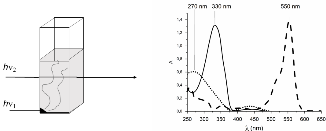
Abb. 6 – links: experimenteller Aufbau um die Farbstofffreisetzung zu verfolgen. – rechts: Absorptionsspektren von trans-Azobenzen (durchgezogene Linie), cis-Azobenzen (gepunktete Linie) und Rhodamin B (gestrichelte Linie).
