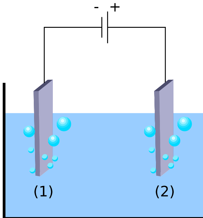
Abb. 1 – Elektrochemische Zelle zur Spaltung von Wasser.
