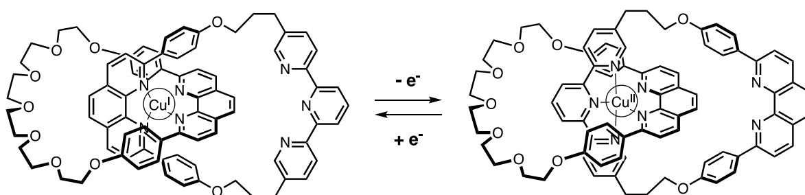
Abb. 1 – Ringkonfigurationen in einem [2]Catenan.
