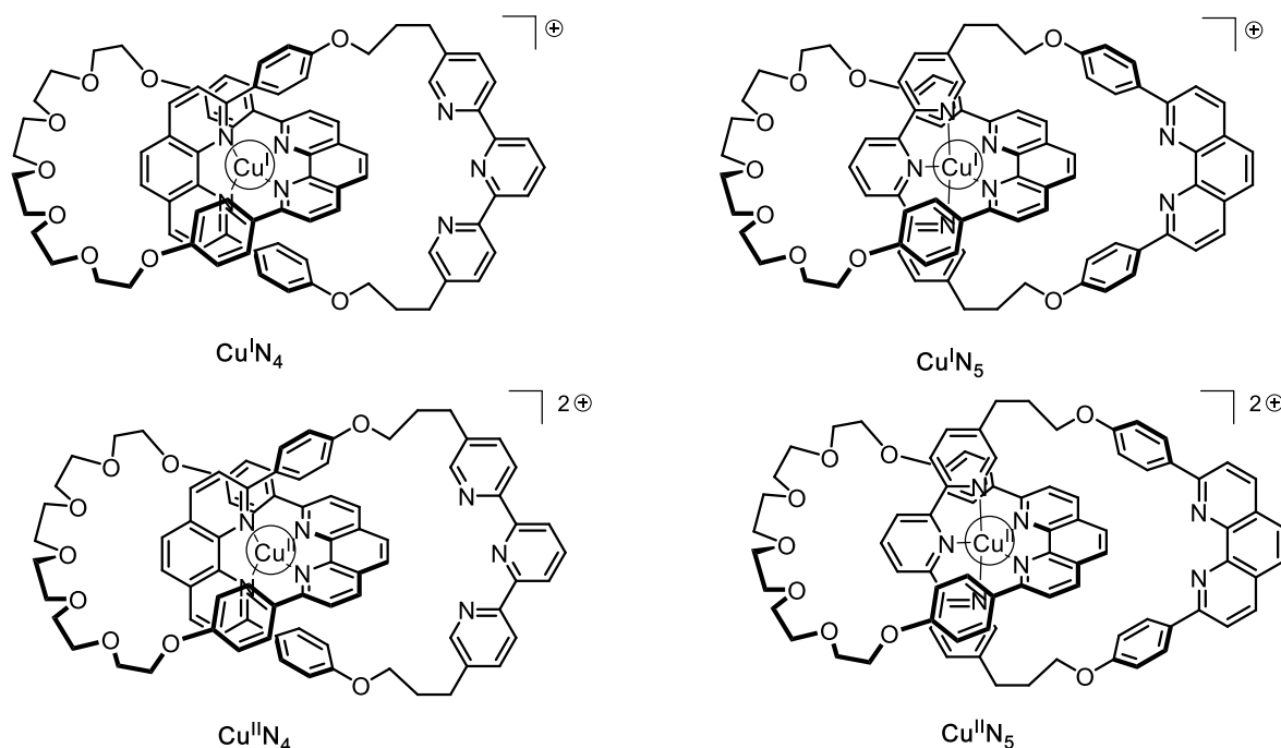
Abb. 2 – Verschiedene Konfigurationen des [2]Catenans L .
