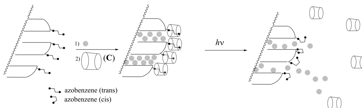
Abb. 5 – Die Dissoziation eines Azobenzene-Cyclodextrin-Einschlusskomplexes wird durch photoinduzierte Isomerisierung eingeleitet und erlaubt Substanzfreisetzung (graue Kugeln).
