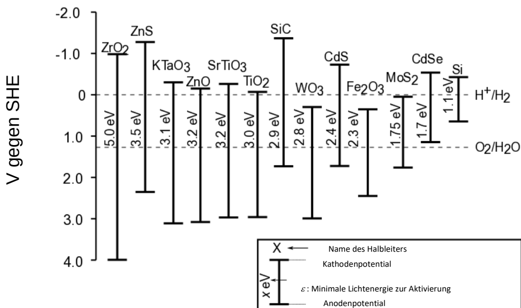
Abb. 2 – Bedingung für die Aktivierung und entsprechende Elektrodenpotentiale für verschiedene Halbleiter. Gestrichelte Linien geben die Potentiale für die Wasseroxidation und -reduktion an. Wasserstoffelektrode (Standard Hydrogen Electrode, SHE).
