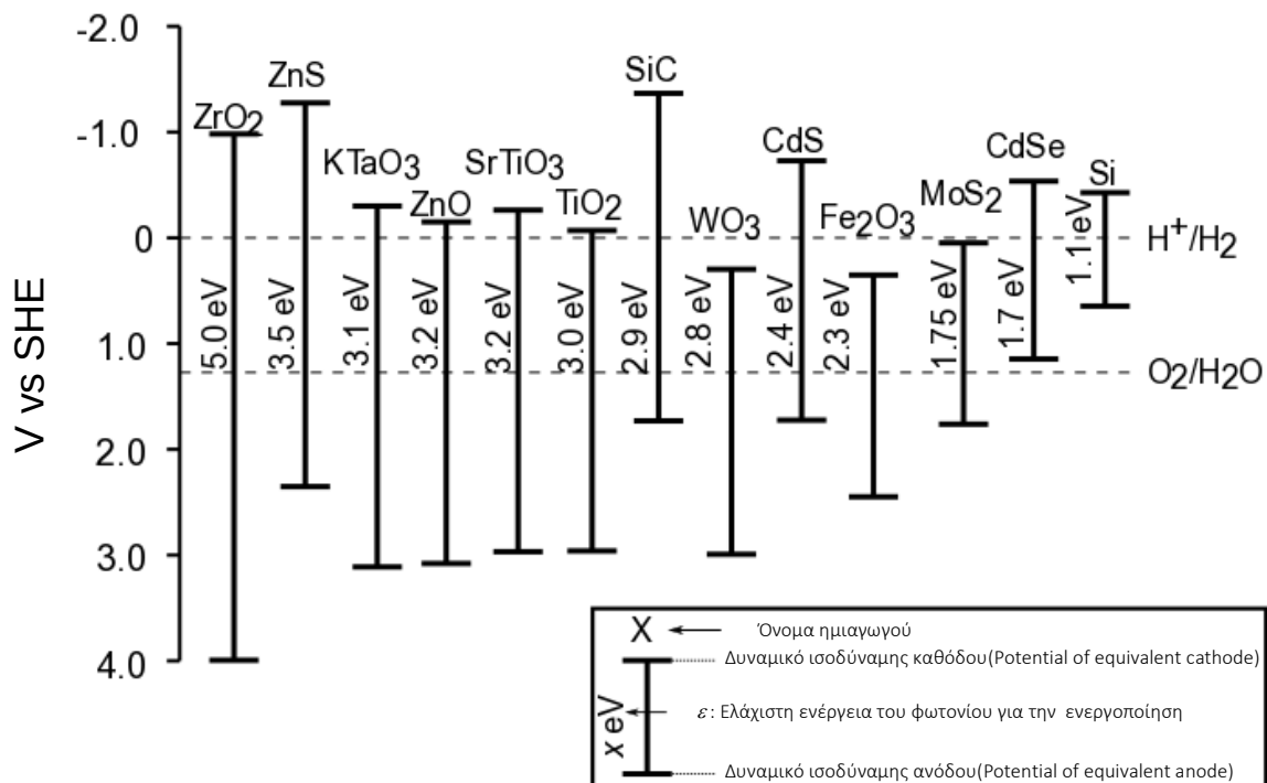
Εικ. 2 – Συνθήκη ενεργοποίησης και δυναμικό ισοδύναμο ηλεκτροδίου για διαφορετικούς ημιαγωγούς.
