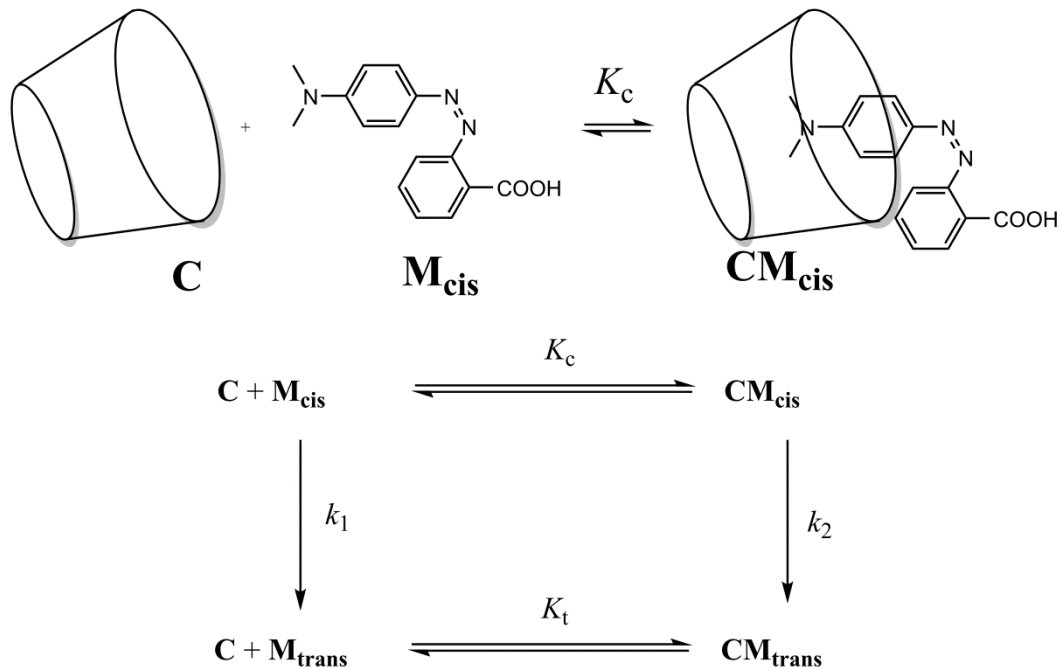
Fig. 4 – Τα στάδια ισομερείωσης της \mathbf{M}_{cis} παρουσία της \mathbf{C} .
