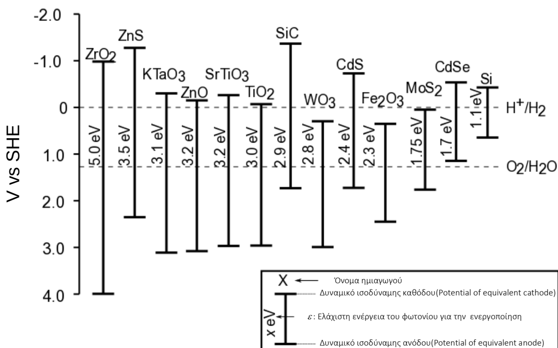
Εικ. 2 – Συνθήκη ενεργοποίησης και δυναμικό ισοδύναμου ηλεκτροδίου για διαφορετικούς ημιαγωγούς.
