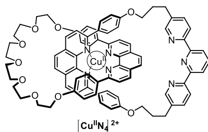
Εικόνα. 2 –οι δομές των συμπλόκων [2]catenane L
