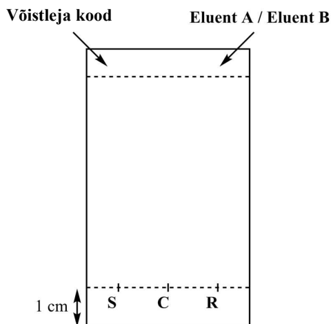
Joonis 3. TLC-plaadi ettevalmistus
