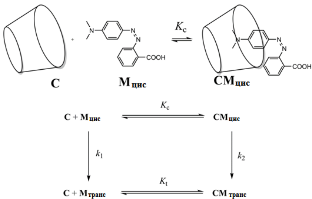
Рис. 4 – Кинетическая схема изомеризации \text{M}_{\text{цис}} в присутствии \text{C} .
