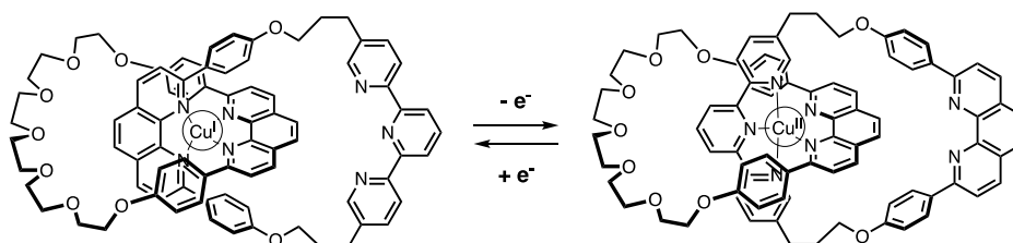
1. attēls – Gredzena multistabilitāte [2]katenānā.
