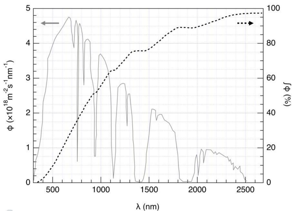
شکل ۳. محور سمت چپ: توزیع طیفی شار (\phi) فوتون‌های خورشیدی. شار فوتون برابر است با تعداد فوتون‌هایی که در واحد زمان به واحد سطح نیم‌رسانا می‌رسند. محور سمت راست و نمودار خط‌چین: شار تجمعی فوتون‌ها (کسری از شار فوتون با طول موج‌های کمتر).
