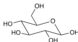
fórmula conformacional
