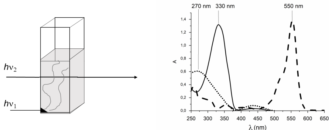
Figuur 6 – Links: Experimentele opstelling voor het volgen van de vrijstelling van de verfstof; rechts: absorptie (=extinctie) spectra van trans-azobenzeen (doorgetrokken lijn), cis-azobenzeen (stippellijn) en rhodamine B (onderbroken lijn).
