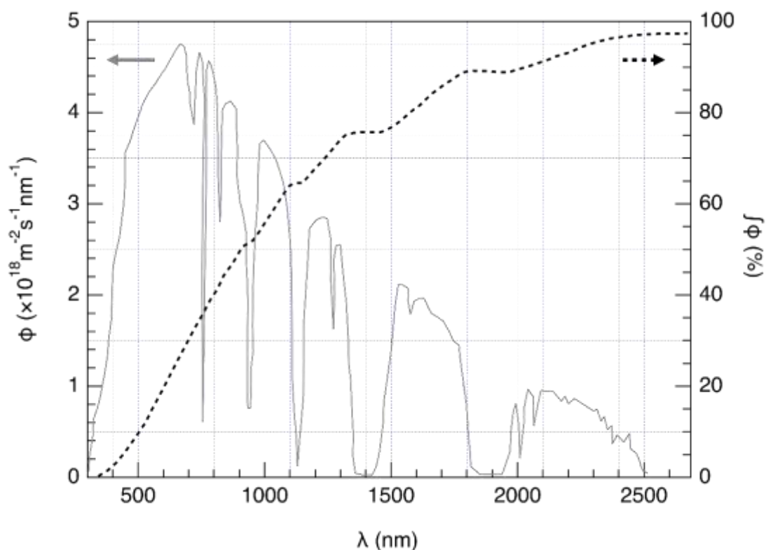
ნახ.3-მარცხენა ღერძი: მზის ფოტონის ნაკადის სპექტრალური განაწილება \Phi . ფოტონების ნაკადი არის დროის ერთეულში ნახევარგამტარის ფართის ერთეულზე დაცემული ფოტონების რაოდენობა. მარჯვენა ღერძი და წყვეტილი ხაზი: კუმულატიური ფოტონების ნაკადი (ე.ი. ყველაზე მოკლე ტალღის სიგრძის ფოტონების ნაკადის ნაწილი)
