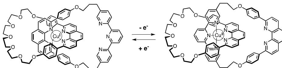
Fig. 1 – Ringbevegelse i en [2]katenan.
