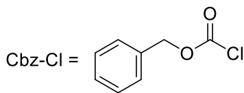
бензилоксикарбонил хлорид
