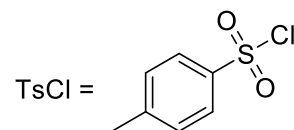
p -толилсульфохлорид
