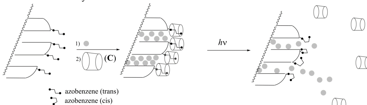
Rys. 5 – Rozszczępienie kompleksu inkluzyjnego azobenzen-cyklodekstryna indukowane przez wywołaną naświetlaniem izomeryzację, co umożliwia uwolnienie barwnika (szare kulki).
